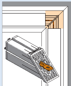
Stabile Eckverbinder im Flügel
